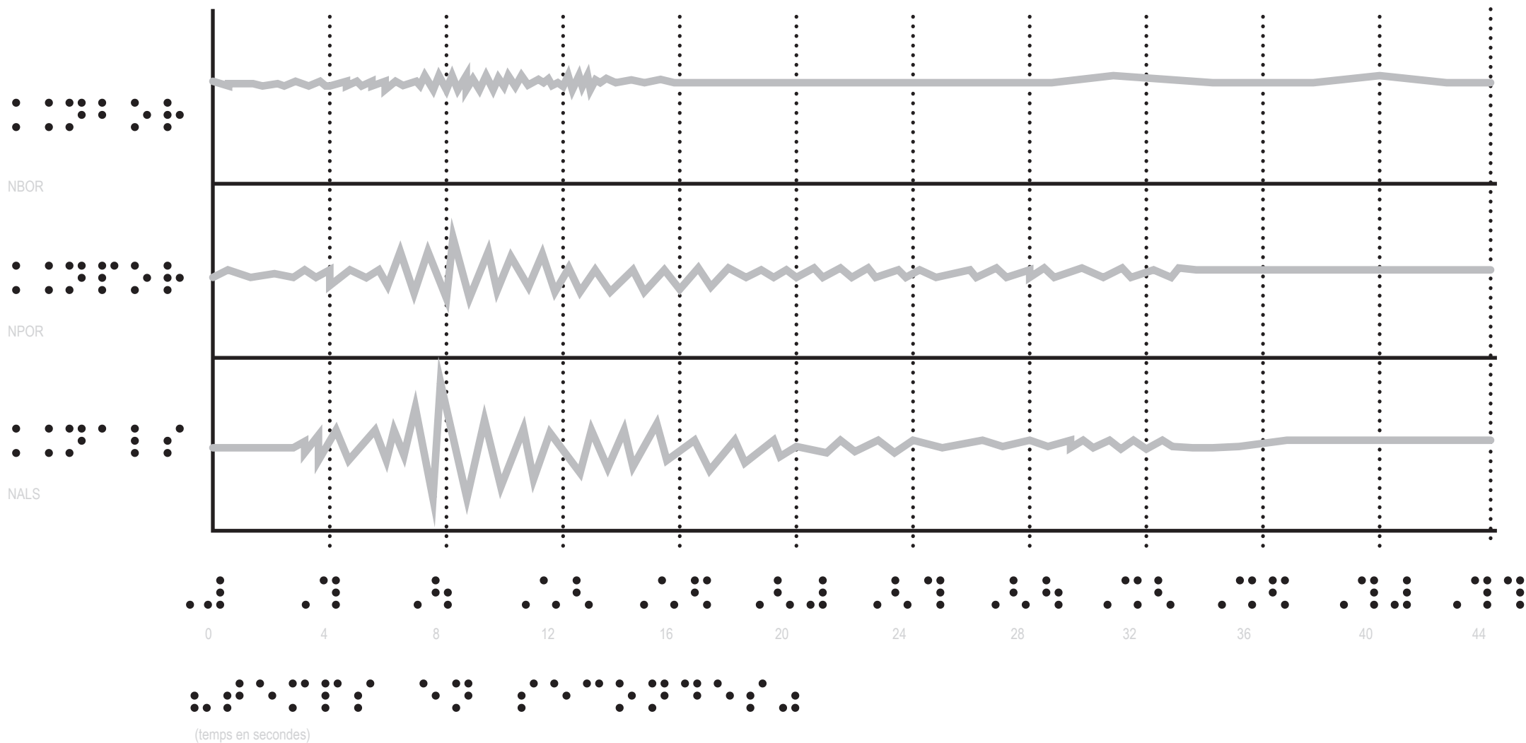
sismogrammes enregistrés dans les stations niçoises localisées (séisme 25 février 2001)
