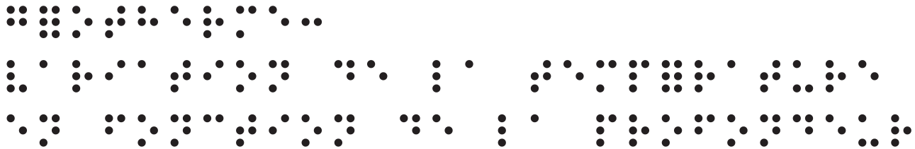
géotherme : variation de la température en fonction de la profondeur
