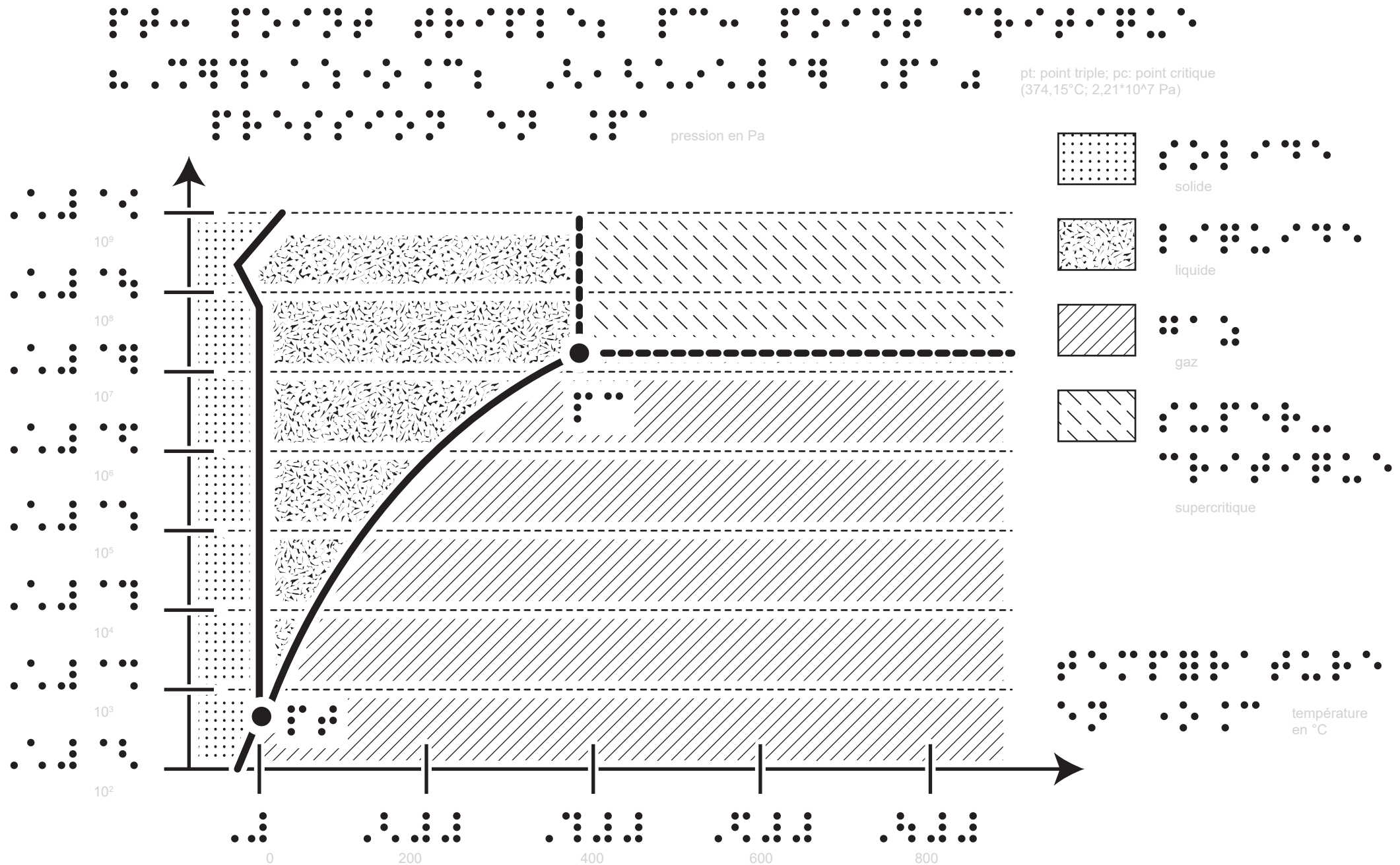
Diagramme d'état de l'eau
