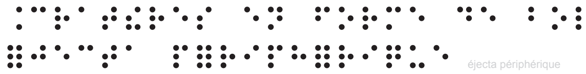
Les cratères
