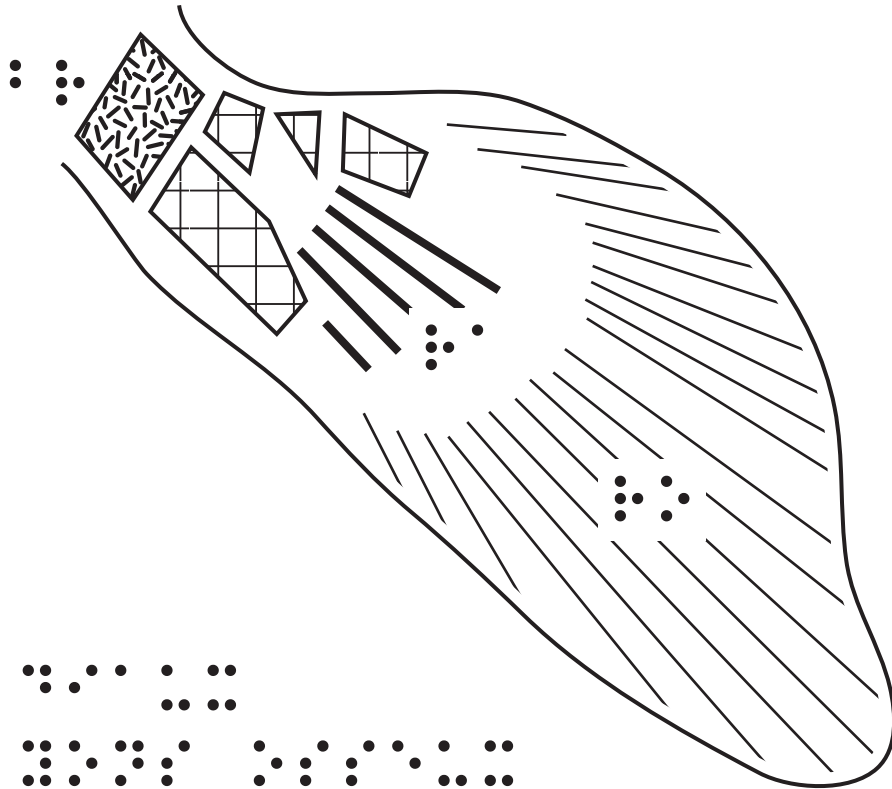
schéma 2 : coelacanth
