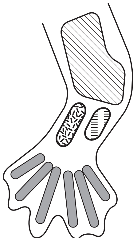
schéma 2 : patte
