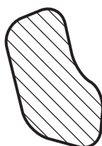
humérus
