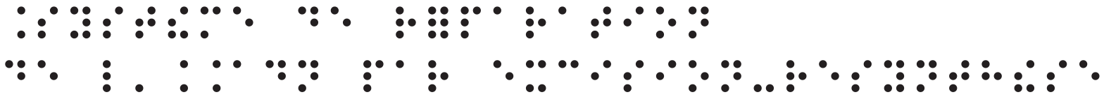
Système de réparation de l'ADN par excision-resynthèse
