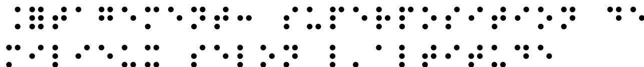
Etagement : superposition de milieux selon l'altitude
